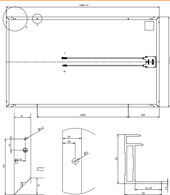
Erdungsbohrung
